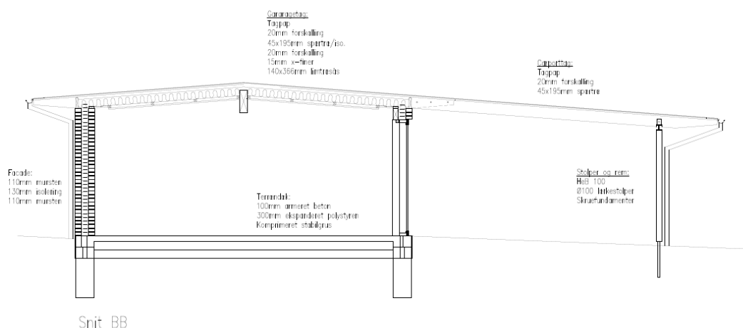
Figur 4. Snit tegning af carport
